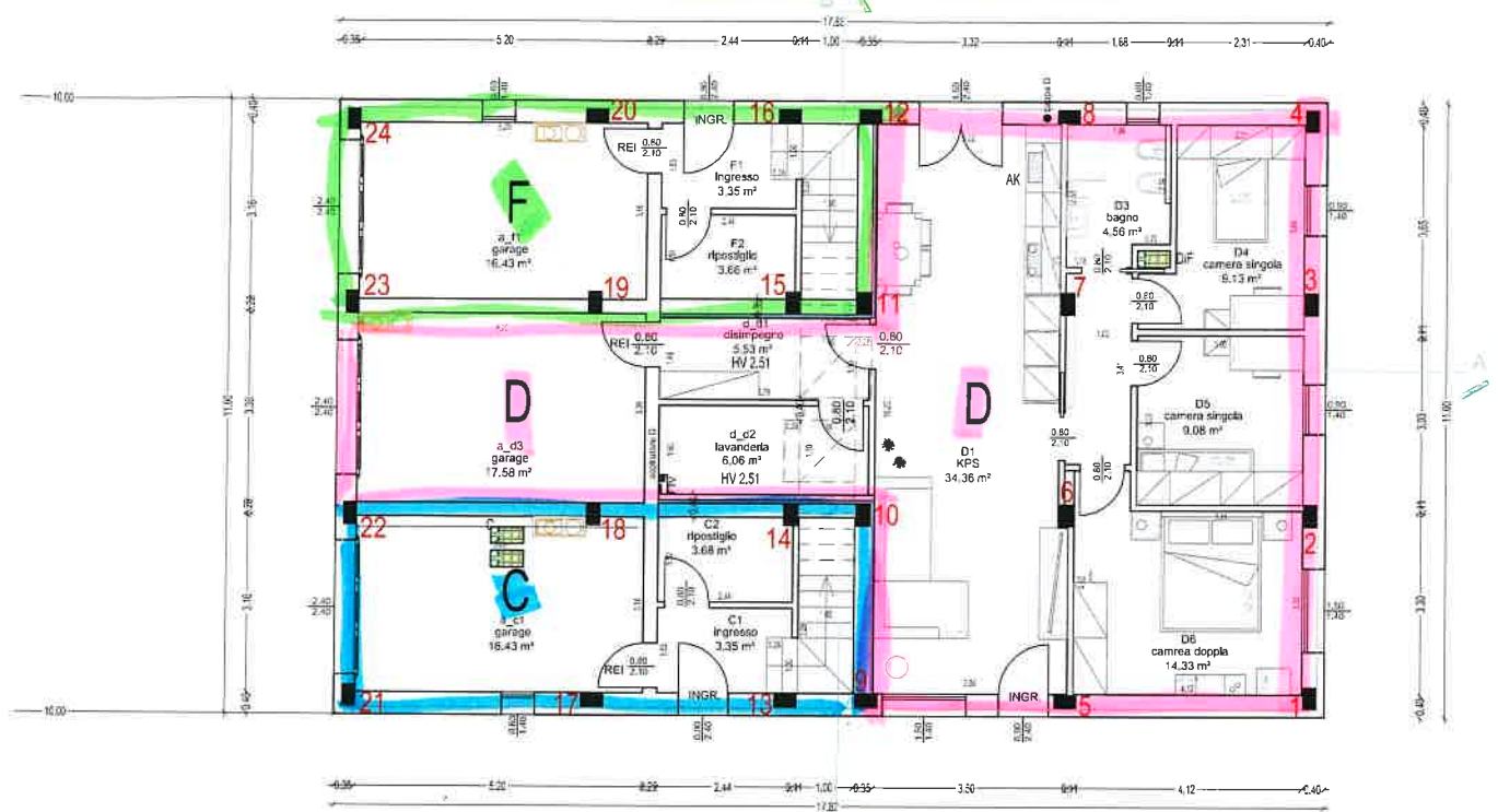
pianta piano terra - DX
