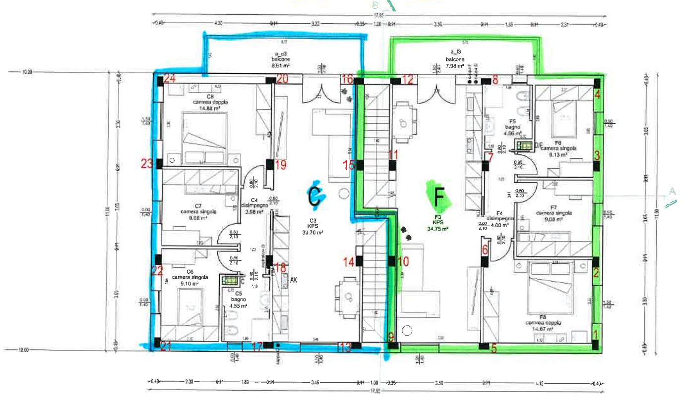
pianta piano primo - DX
