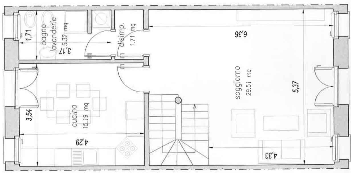
piano terra scala 1:50
