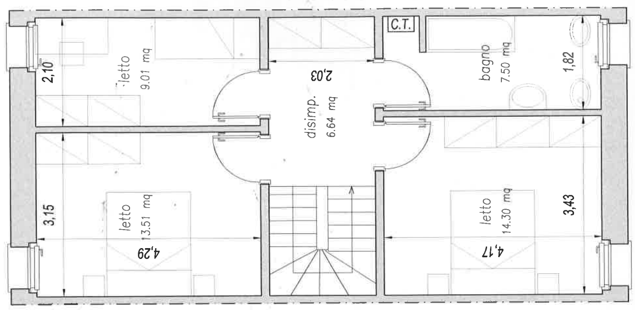
piano primo scala 1:50
